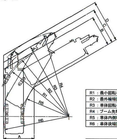
2輪ステアリングで右折する場合
